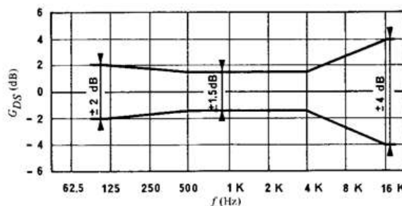
Сл. 1 - Дозволени толеранции за амплитудно-фреквенциската карактеристика на студиските мониториншки слушалки (според ITU препораката – ITU-R BS. 708)
