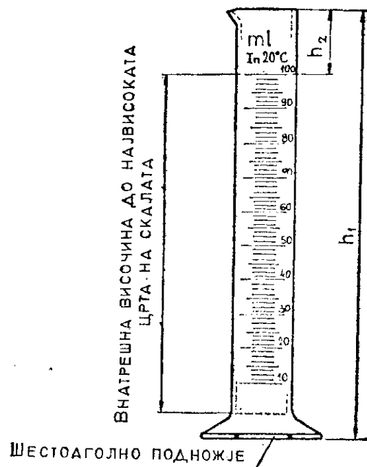
Цртеж бр. 1. Општ изглед на цилиндар со клун за излевање на течност
