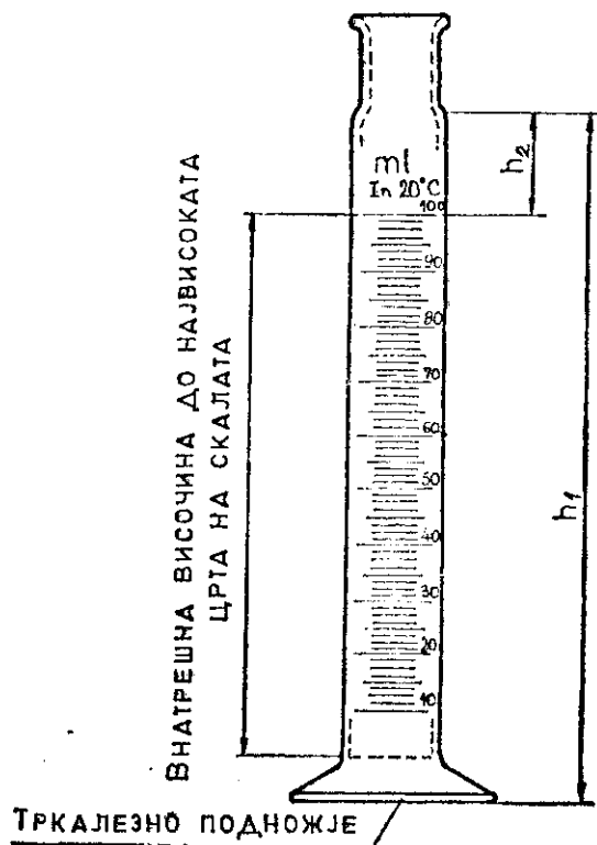
Цртеж бр. 2. Општ изглед на цилиндар со стеснет врат
