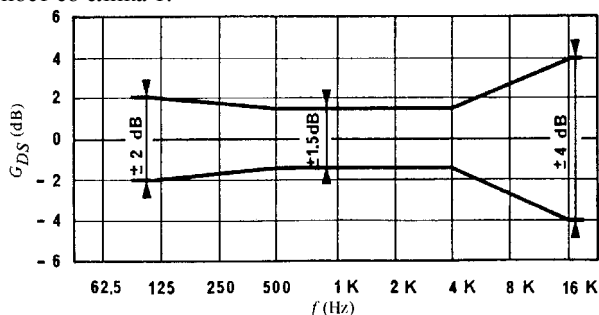
сл. 1 - Дозволени толеранции за амплитудно-фреквенциската карактеристика на студиските мониторинг слушалки (според ИТУ препораката - ITU-R Recommendation BS.708 [3])
