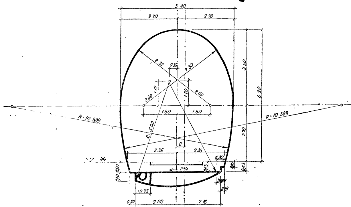
Слика 3 Светол профил на едноколосечен тунел
