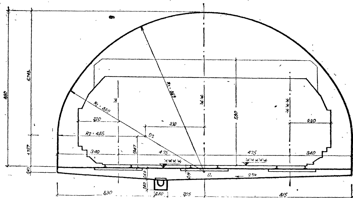
Слика 5. Светол профил на триколосечен тунел
