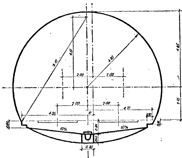
Слика 4. Светол профил на двоколосечен тунел
