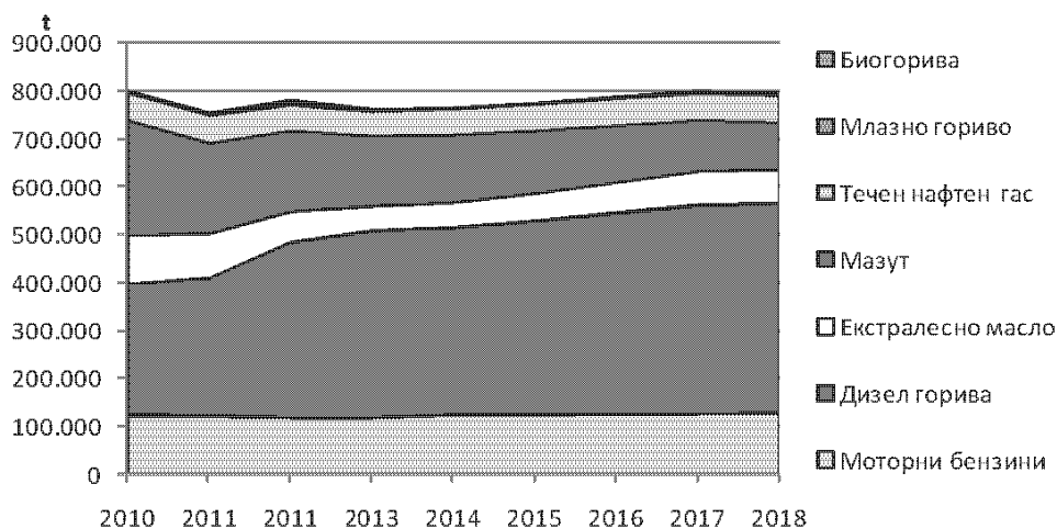
Слика 2.9 Потрошувачка на нафтени деривати во периодот од 2010 до 2018 година
