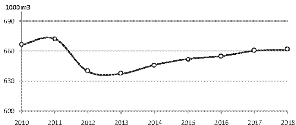
Слика 2.12 Потрошувачка на огревно дрво во периодот од 2010 до 2018 година
