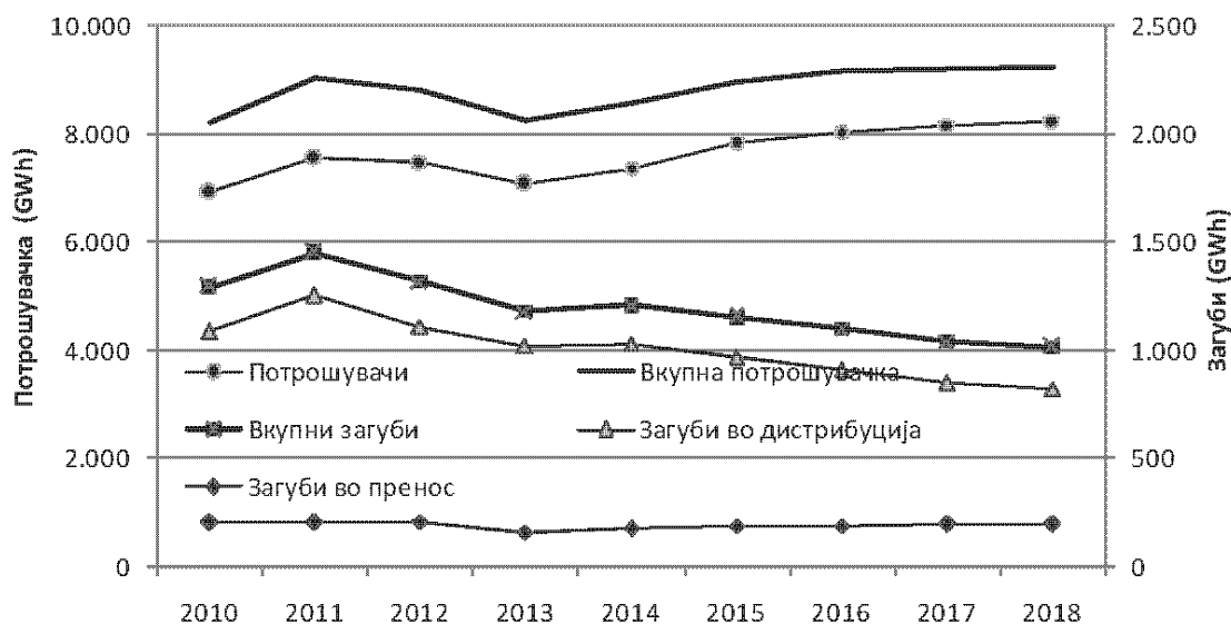
Слика 2.6 Потрошувачка на електрична енергија и загуби во во периодот од 2010 до 2018 година
