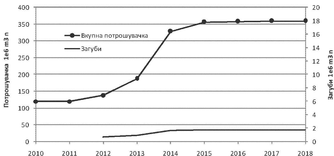
Слика 2.8 Потрошувачка на природен гас и загуби во периодот од 2010 до 2018 година
