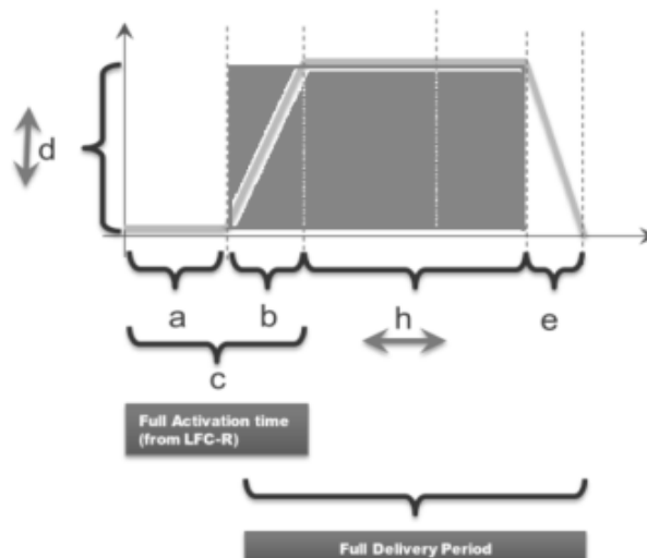
Слика 3: Количина на активирана mFRR балансна енергија (сино обоен правоаголник) ( Full Activation time = вкупно време на активација (од LFC-R); Full Delivery Period = вкупно време на испорака)
