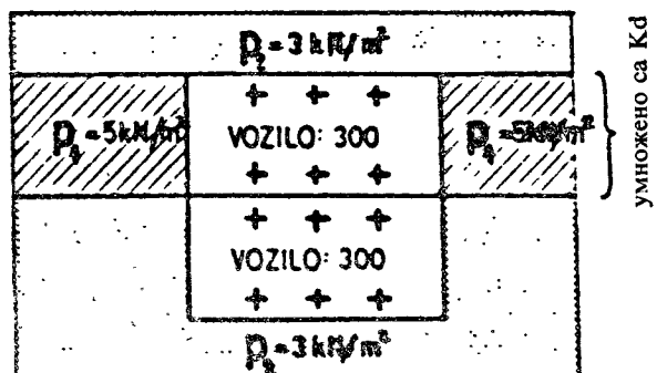
Слика 2 – Рачунске шеме оптерећења
