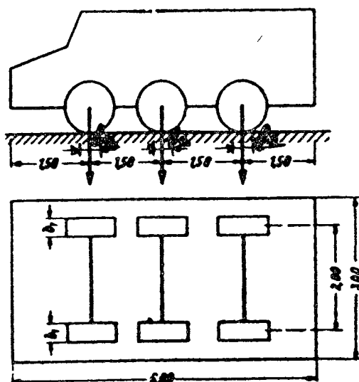
Слика 1 – Типско возило V 600 или V 300
