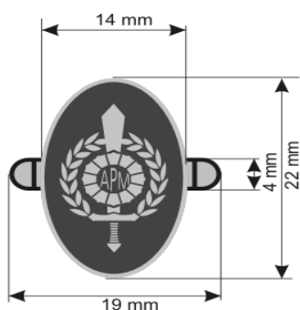
копче за манжетна од кошула за службена униформа
