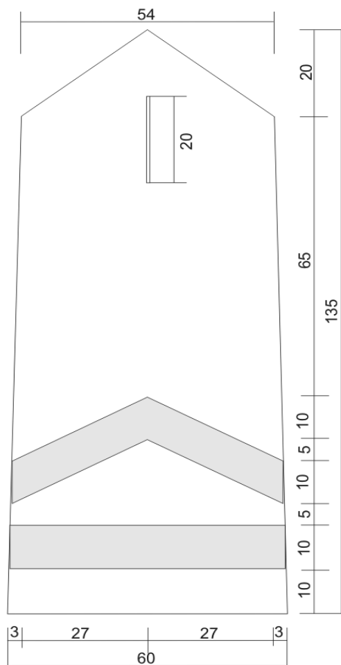
Еполети за чин за службена униформа
