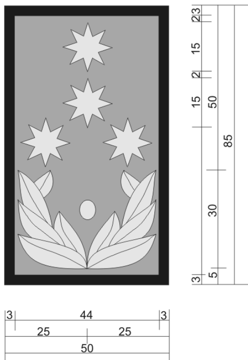
Ознака за чин за военотеренска униформа
