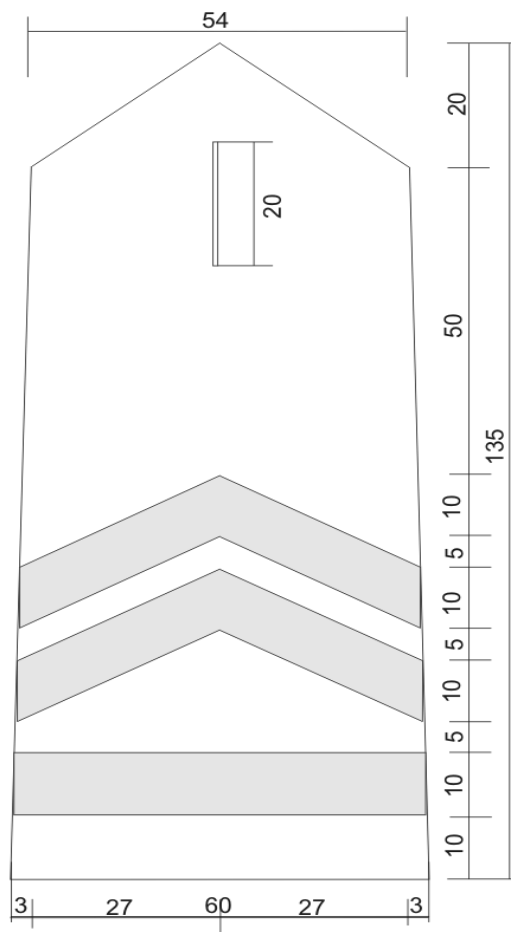
Еполети за чин за службена униформа
